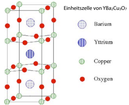
Abbildung 9.14: Typische Struktur eines Hochtemperatur-Supraleiters.
