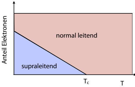
Abbildung 9.22: Das Modell der zwei Flüssigkeiten.
