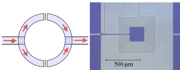
Abbildung 9.42: Schematischer Aufbau und Bild eins SQUIDs.
