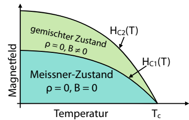
Abbildung 9.11: Unterschiedliche Phasen bei einem Typ II Supraleiter.
