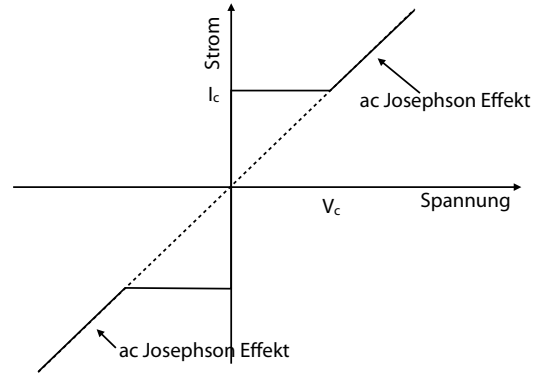
Abbildung 9.39: Strom-Spannungs Kurve bei einem Josephson Kontakt.
