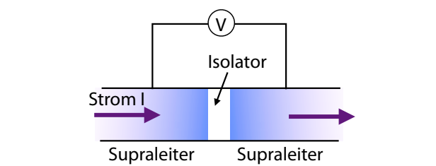
Abbildung 9.36: Tunnelkontakt zwischen zwei Supraleitern.
