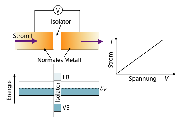
Abbildung 9.34: Tunnelkontakt zwischen zwei Normalleitern.
