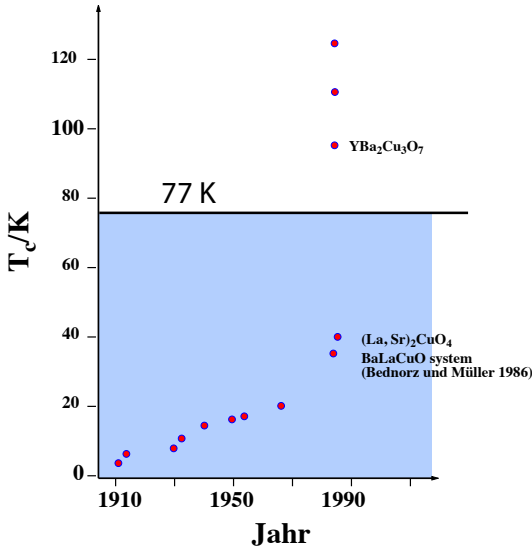
Abbildung 9.20: Maximale kritische Temperatur als Funktion der Zeit.
