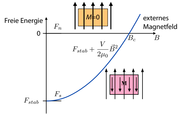
Abbildung 9.21: Energie des normalleitenden Zustandes ( F_n ) und des supraleitenden Zustandes ( F_s ) als Funktion der Stärke des externen Magnetfeldes.
