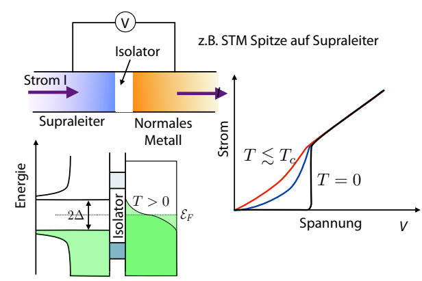
Abbildung 9.35: Tunnelkontakt zwischen Supraleiter und Normalleiter.
