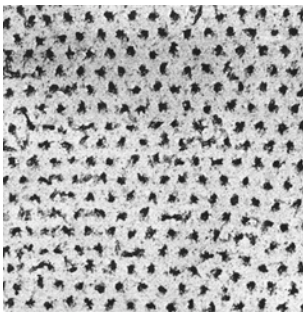
Abbildung 9.13: Hexagonales Gitter aus Flussquanten.
