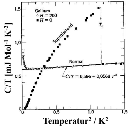
Abbildung 9.17: Spezifische Wärme von Gallium (links) und der elektronische Beitrag (rechts).
