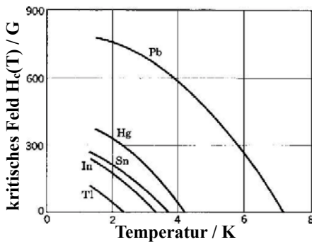
Abbildung 9.9: Temperaturabhängigkeit des kritischen Feldes bei Typ I Supraleiter.
