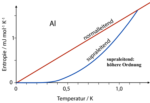
Abbildung 9.15: Temperaturabhängige Entropie von Aluminium.
