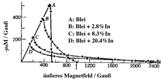
Abbildung 9.10: Magnetisierung als Funktion der Temperatur für Blei mit unterschiedlicher Dotierung.
