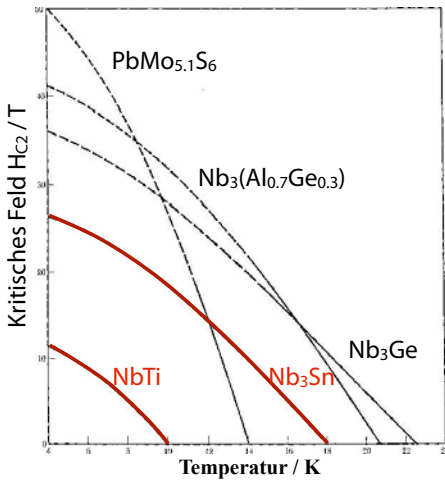
Abbildung 9.12: Temperaturabhängigkeit des oberen kritischen Feldes bei Typ II Supraleitern.
