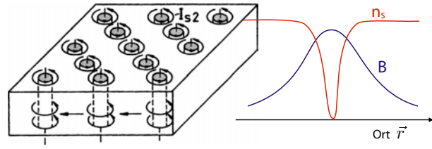
Abbildung 9.25: Verlauf des Ordnungsparameters n_s in der Nähe eines Fluss Schlauches in einem Typ II Supraleiter.
