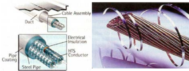
Abbildung 9.32: Supraleitende Drähte.
