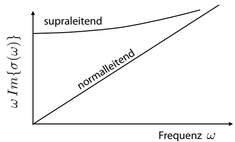
Abbildung 9.33: Dispersion der Leitfähigkeit.
