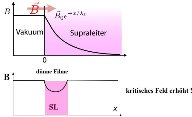
Abbildung 9.23: Eindringen des Magnetfeldes in Volumensupraleiter und in dünne Schichten.
