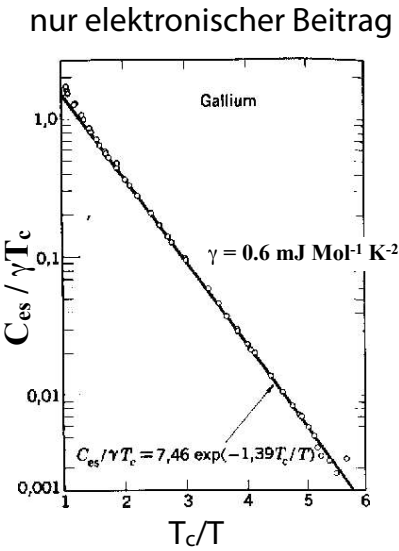
Abbildung 9.18: Spezifische Wärme von Gallium (links) und der elektronische Beitrag (rechts).
