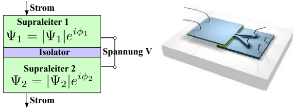
Abbildung 9.38: Josephson-Kontakt.
