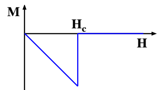
Abbildung 9.5: Magnetisierung als Funktion des äußeren Feldes.
