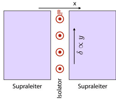
Abbildung 9.40: Effekt eines Magnetfeldes auf die Phasendifferenz eines Josephson Kontaktes.
