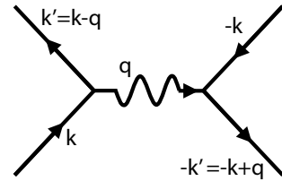
Abbildung 9.29: Wechselwirkung durch Emission und Absorption eines Phonons.
