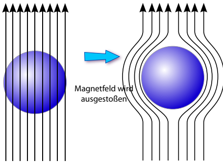
Abbildung 9.6: Meissner-Effekt: Ein Supraleiter ist ein perfekter Diamagnet.
