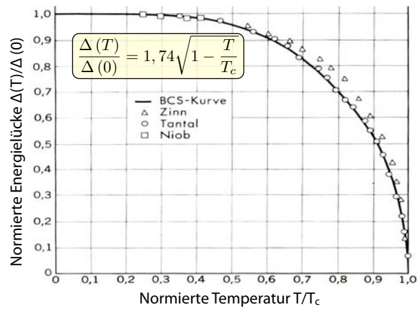
Abbildung 9.31: Normierte Energielücke als Funktion der Temperatur.
