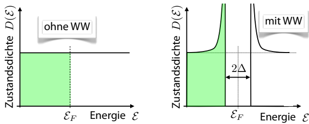
Abbildung 9.30: Energielücke an der Fermikante.
