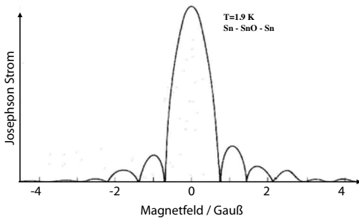
Abbildung 9.41: Abhängigkeit des Josephson Stroms von der Flussdichte.
