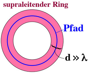
Abbildung 9.27: Geschlossener Pfad in einem supraleitenden Ring.
