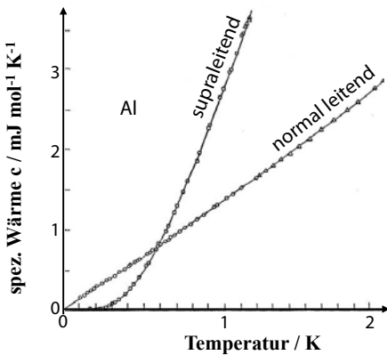
Abbildung 9.16: Temperaturabhängige spezifische Wärme von Aluminium.
