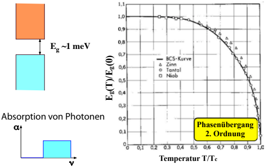
Abbildung 9.19: Energielücke, Temperaturabhängigkeit und Absorptionsspektrum.
