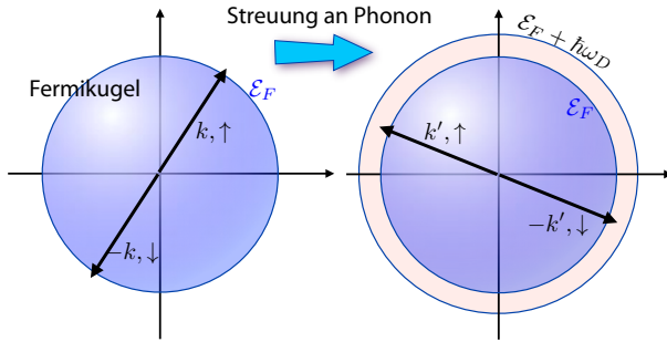
Abbildung 9.28: Streuung eines Elektronenpaares mit einem Phonon.
