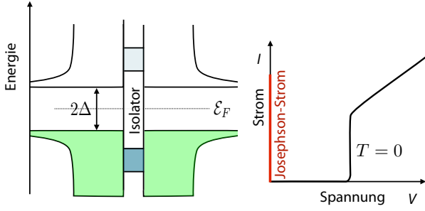
Abbildung 9.37: Zustandsdichten an einem Josephson Kontakt und Strom-Spannungs Kennlinie.
