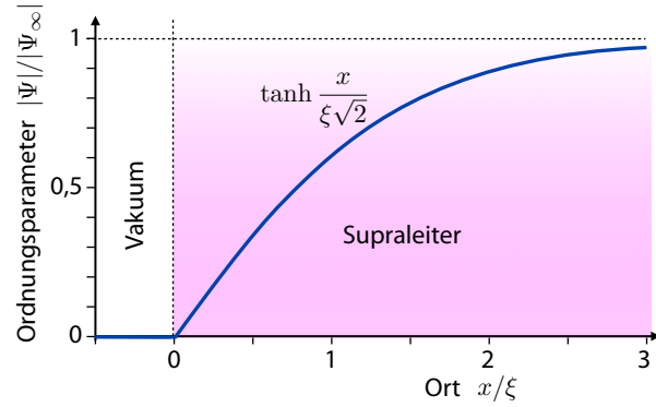
Abbildung 9.26: Anstieg des Ginsburg-Landau Ordnungsparameters von der Grenzfläche bei x = 0 .
